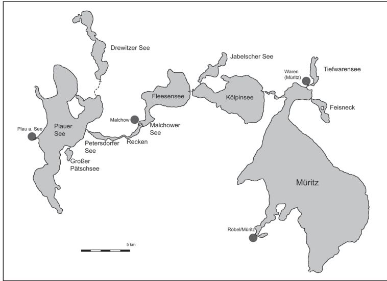
Abb. 2: Das Untersuchungsgebiet Mecklenburgische Oberseen
