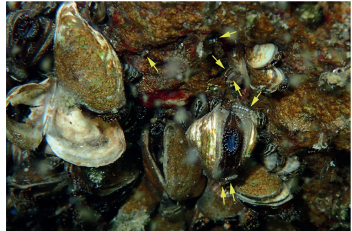
Abb. 9: Dreissena bugensis bietet optimales Habitat für Dikerogammarus villosus (Sowinsky, 1894) und Echinogammarus ischnus (Stebbing, 1899), (Pfeile: Dikerogammarus villosus (Sowinsky, 1894))
