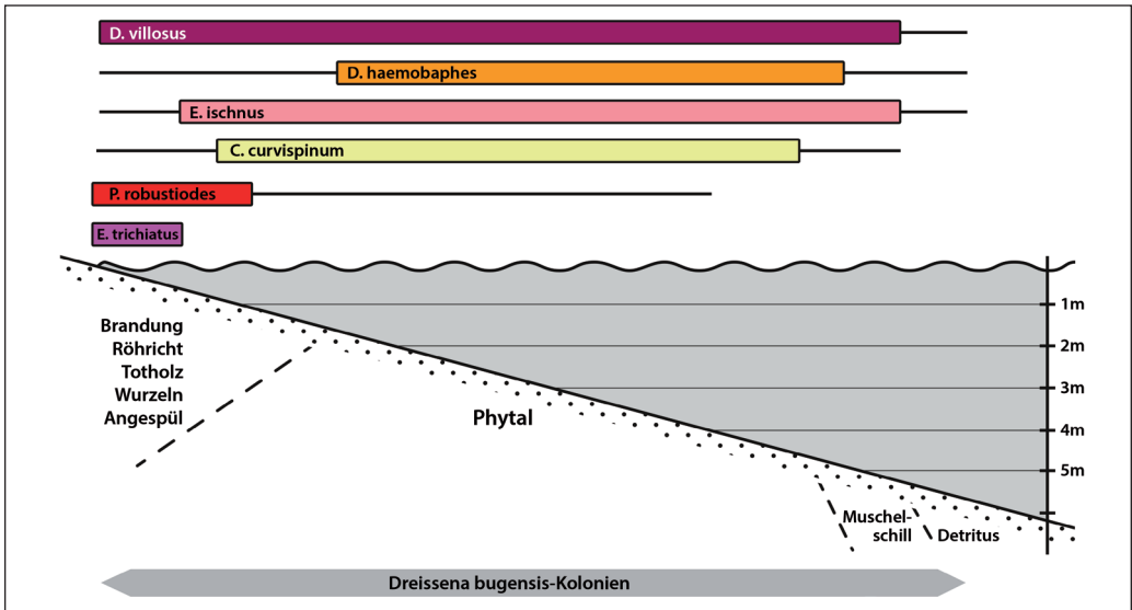
Abb. 4: Tiefenverteilung der Arten in den großen Seen (Müritz, Kölpinsee, Fleesensee, Plauer See sowie deren Verbindungen)
