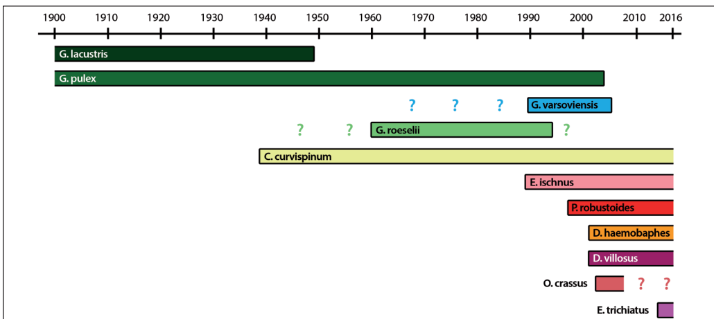
Abb. 5: Zeittafel der Funddaten von Amphipoden von 1901 bis 2016
