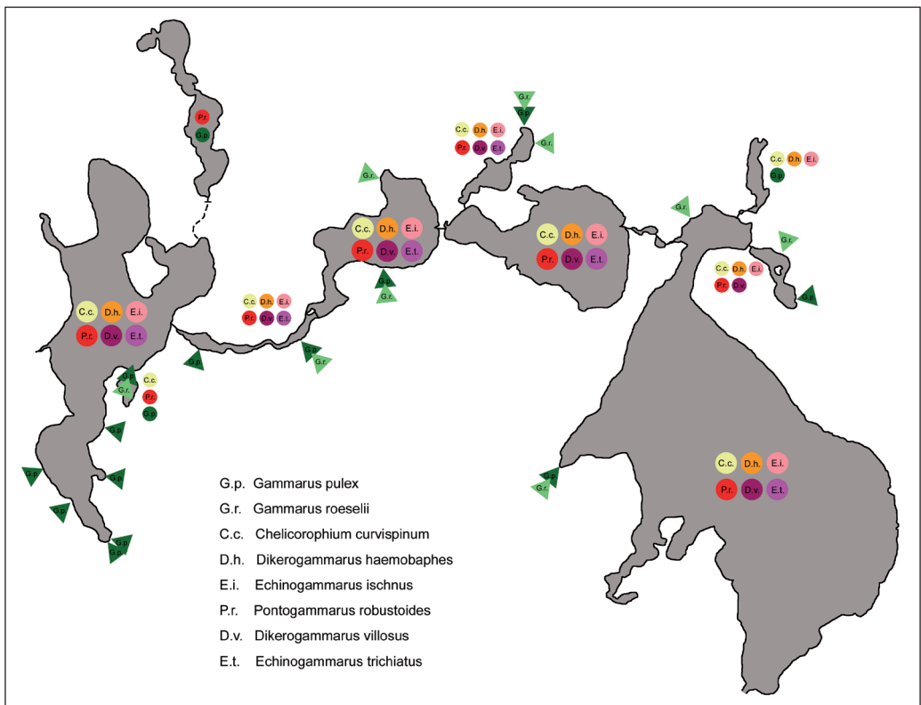
Abb. 3: Verbreitung der Amphipodenarten 2014–2016 im Untersuchungsgebiet (ohne Synurella ambulans (F. Müller, 1846))
